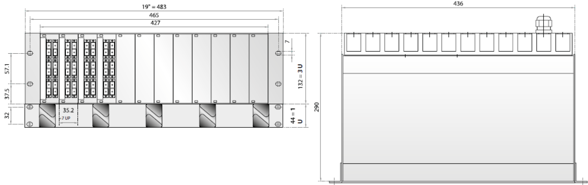
VUE DE DOS : PRESSE-ÉTOUPE PG DANS L'ESPACE DE LOVAGE ARRIÈRE 1 U
