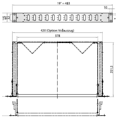
ABMESSUNGEN 1 HE
