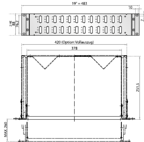
ABMESSUNGEN 2 HE
