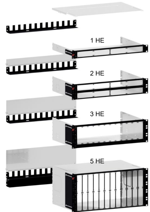
1 HE 1/4 Blind-TFP RAL9005 schwarz Bestellnummer: 170A0001
